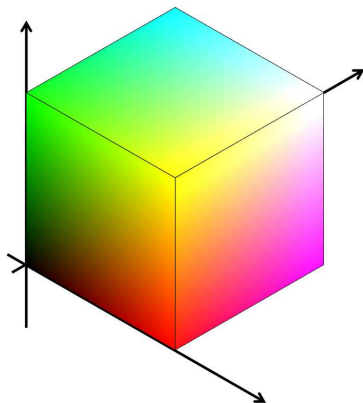
RGB
